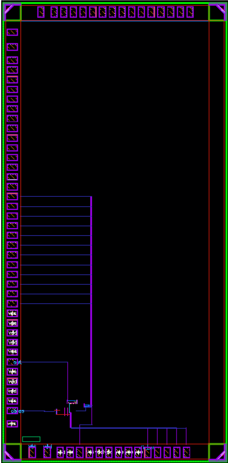
[전체 Die layout]
