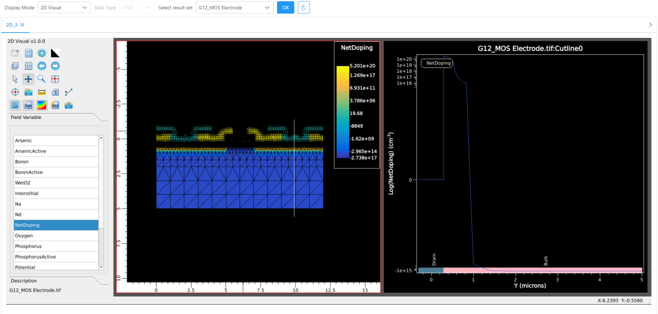
Simulation 결과에 대한 Window Tab 방식의 Displaying 지원
