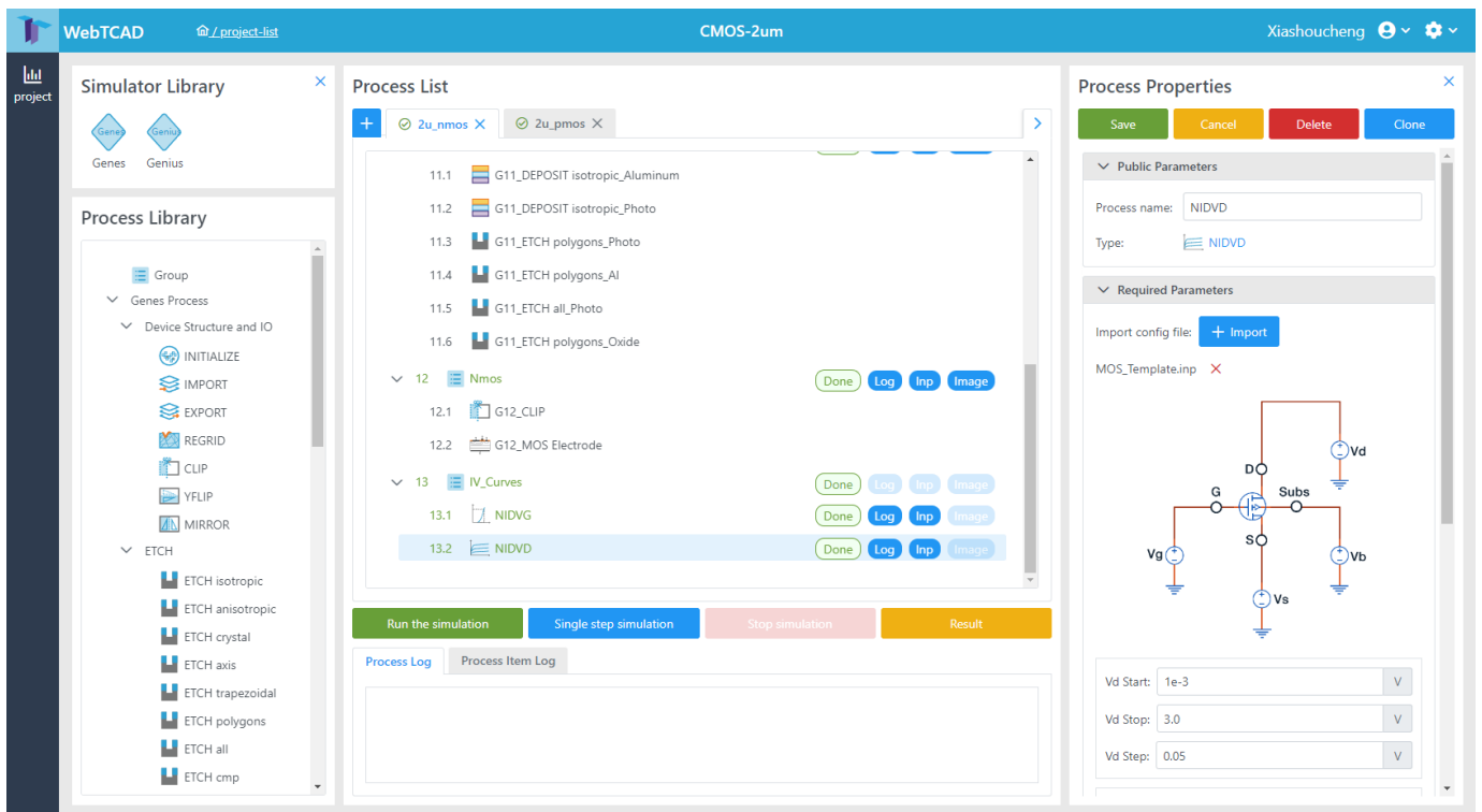
Cloud 기반 동작을 통해 Web에서의 간편 Setup 가능
