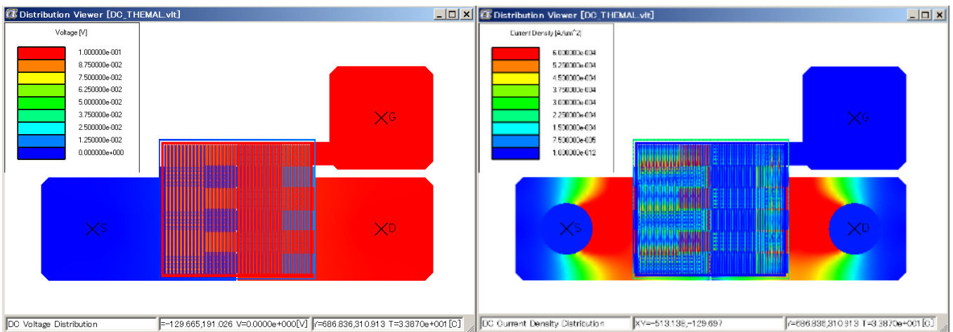
DC Analysis 에 대한 Layout 기반 Contour 분석 제공 (Voltage Distribution / Current Density)
