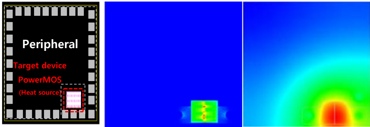
Thermal Analysis 결과에 대한 Distribution / Density 표시 등의 분석 기능 제공 ( W/m^3 )
