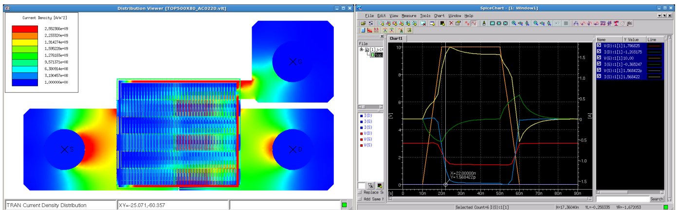
Transient Analysis 에 대한 Layout 기반 Contour 분석 제공
